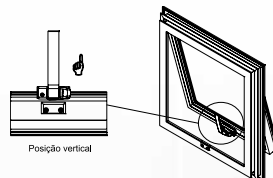
Posição do fecho quando a folha aberta
