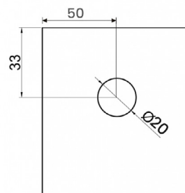
1126M - Mini carrinho roldana meia cana
