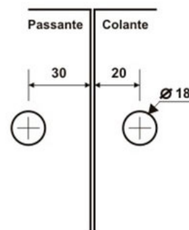
1321 - Suporte inferior para união 2 vidros 90°
