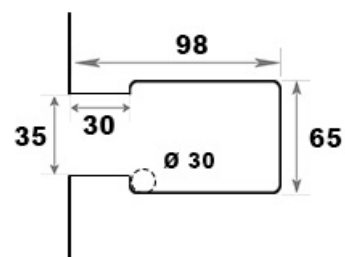
1128B - Dobradiça lateral de canto para portas em arco
