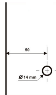
1671 - Puxador para janela simples que permite transpasse 1671MD - Puxador para janela duplo que permite transpasse
