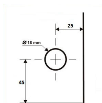
1800AS - Trinco de pressão para janela de correr
