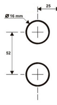
1510MP - Mini fechadura de pressão para janela correr
