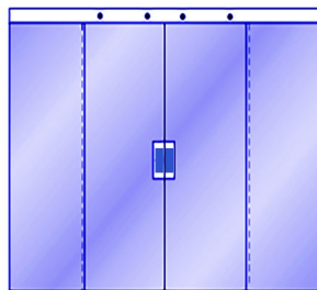
V1570 - Bate-fecha central V/V modelo Vialtec com tranca
