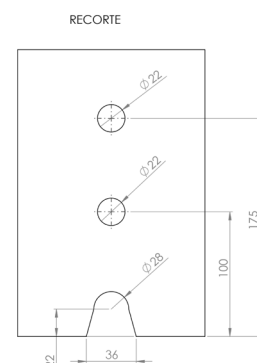
1103R - Dobradiça vertical inferior para mola
