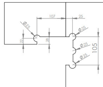
1209PG - Facção grande lateral para bandeira
