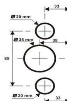
1510XC - Fechadura para porta de correr com desvio de perfil
