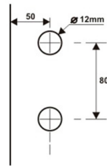
1670 - Puxador de 1 lado porta correr 80 entre furos 1670D - Puxador de 2 lados porta correr 80 entre furos
