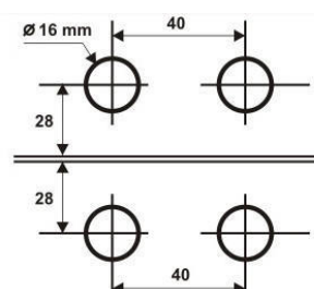
1132 - Dobradiça maxim-ar v/a com 40mm entre furos
