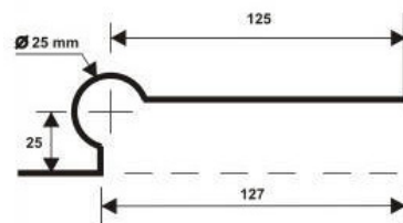
1102G - Dobradiça pivotante inferior grande
