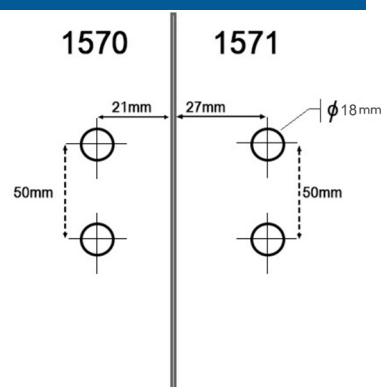
V1570 90° - Bate-fecha de canto 90° V/V
