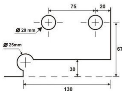
1103G - Dobradiça grande inferior para mola
