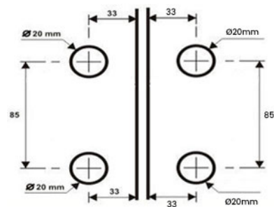
1570G - Bate-fecha central v/v p/janela grande furação Blindex * sem miolo*
