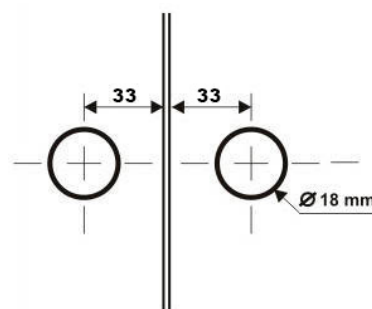
1570FG - Bate-fecha GIROFLECK V/A para janela
