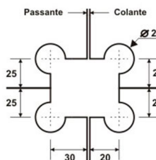
1319 - Suporte para união de 4 vidros a 90°
