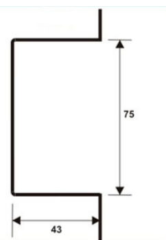
1504 - Contra fechadura sem aba para 1520
