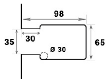
1128A - Dobradiça lateral para portas em arco
