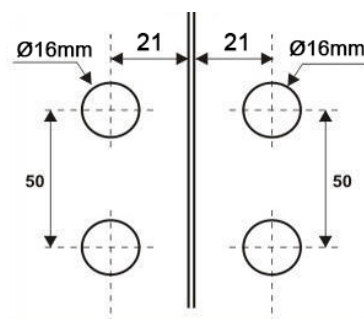
V1570 90° - Bate-fecha de canto 90° V/V
