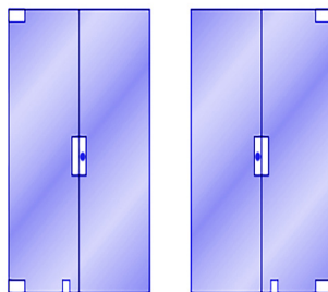
1504AX - Batedeira em alvenaria para 1520X
